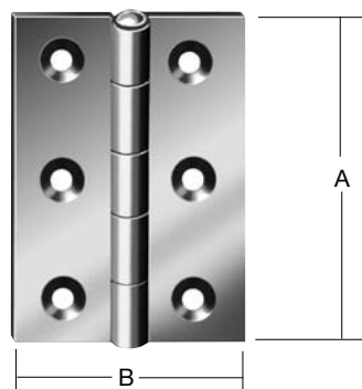
Gerollte halbbreite Scharniere DIN 7954 B mit vernietetem Eisenstift
