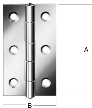
Gerollte schmale Scharniere DIN 7954 A mit vernietetem Eisenstift
