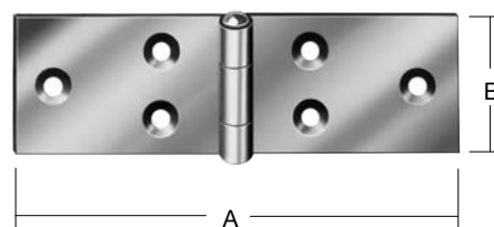
Gerollte breite Tischbänder DIN 7957 mit vernietetem Eisenstift
