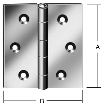
Gerollte kántige Scharniere DIN 7954 C mit vernietetem Eisenstift
