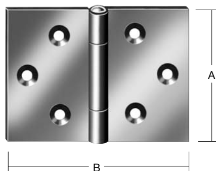
Gerollte breite Scharniere DIN 7954 D mit vernietetem Eisenstift
