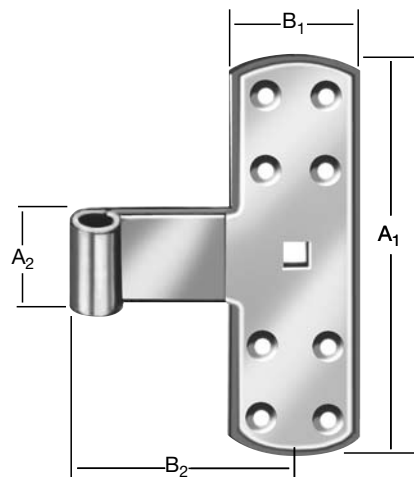
Kreuzbänder für Dorn-Ø 13 mm
