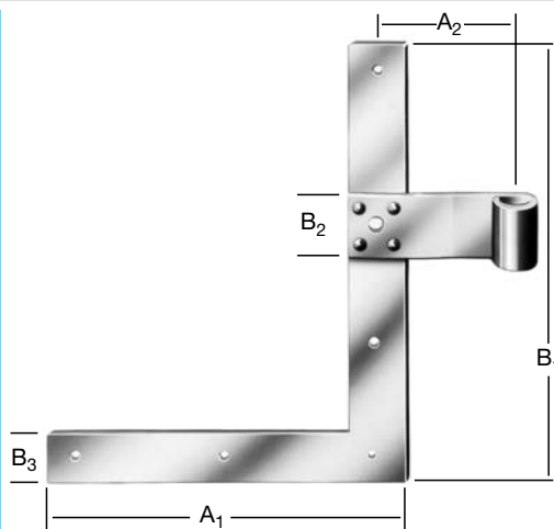
Fensterladen-Winkelbänder für Dorn-Ø 13 mm
