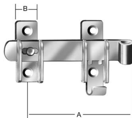
Sicherheits-Schlagladen-Überwürfe mit Griffmulde
